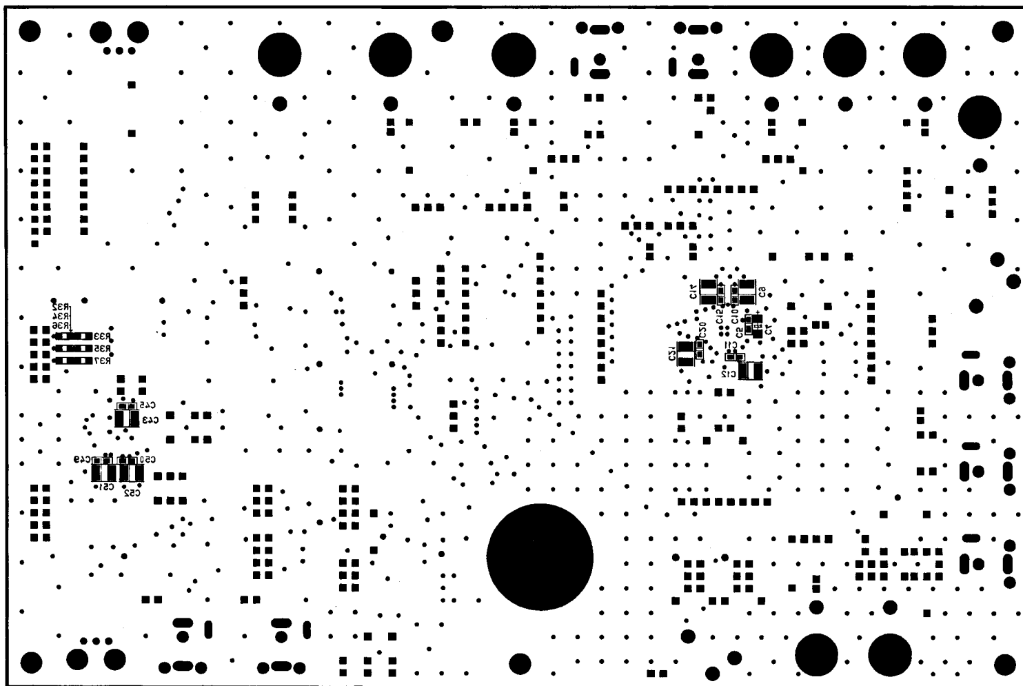
AKD4632-A L2_SILK
