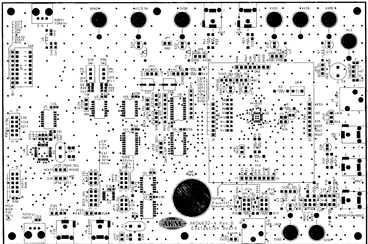
AKD4632-A L1_SILK
