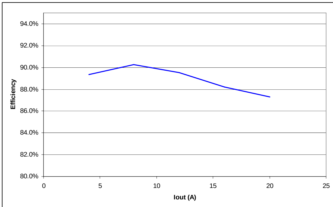
20 Amp Output
