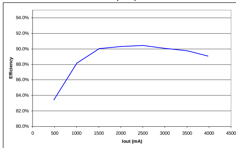
4 Amp Output
