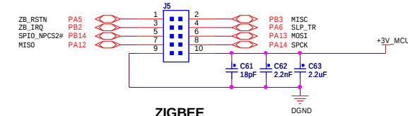
ZIGBEE
