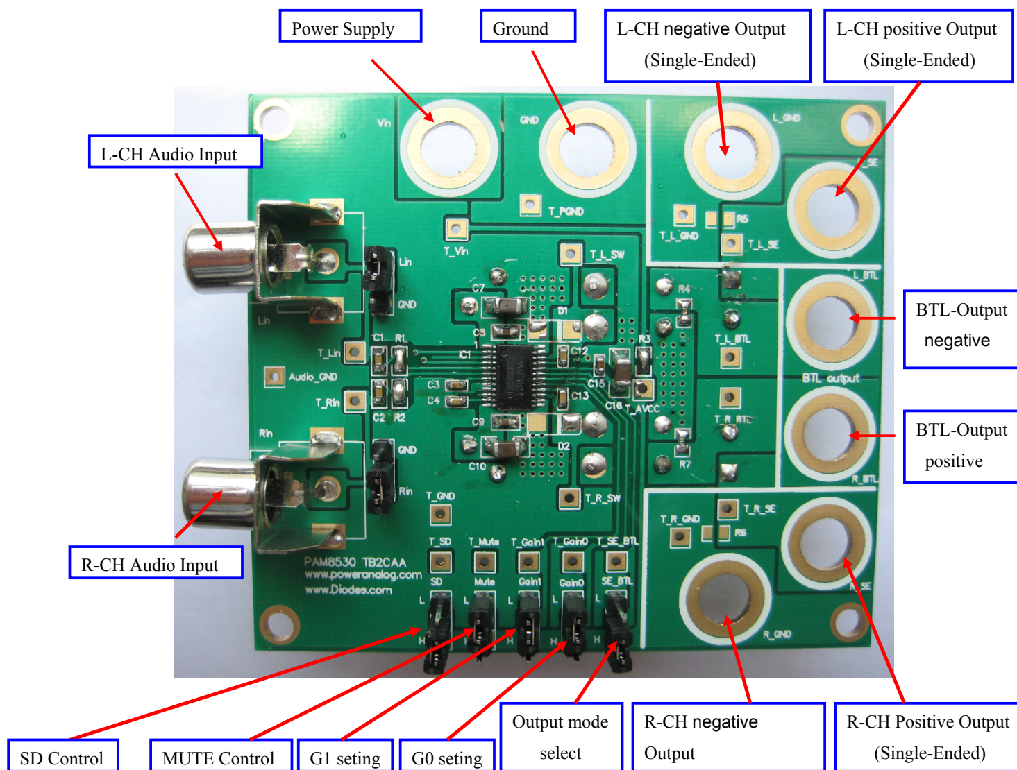
Top Layer
