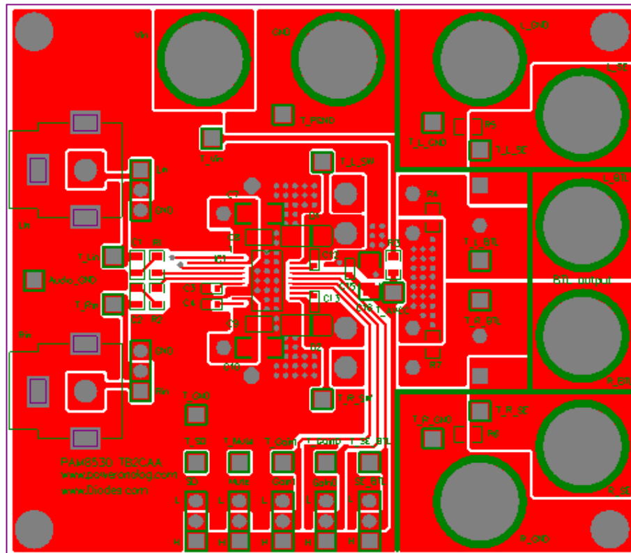
Top layer
