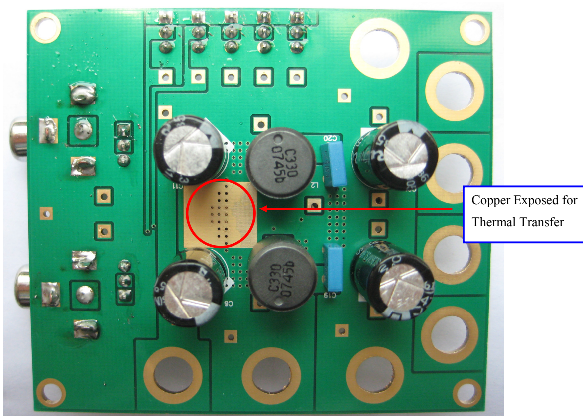
Bottom Layer
