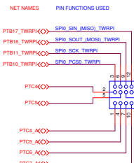
SPI0 TWRPI/TWR_ELEV Select
