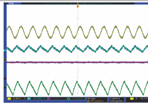
CH1: V_{(SUPPLY)} CH2: V_{(REF)} CH3: V_{(IOUT8)} CH4: I_{(IOUT8)} I_{(IOUT8)} = 35 \text{ mA}
