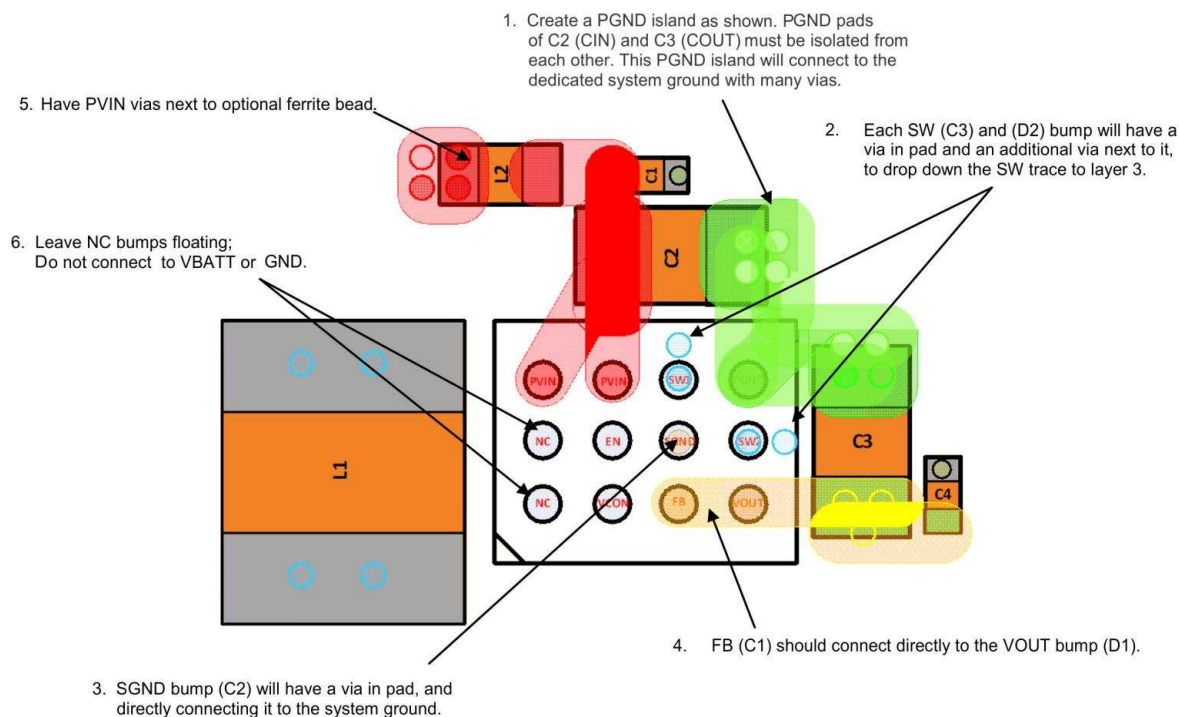
Figure 18. Top Layer
